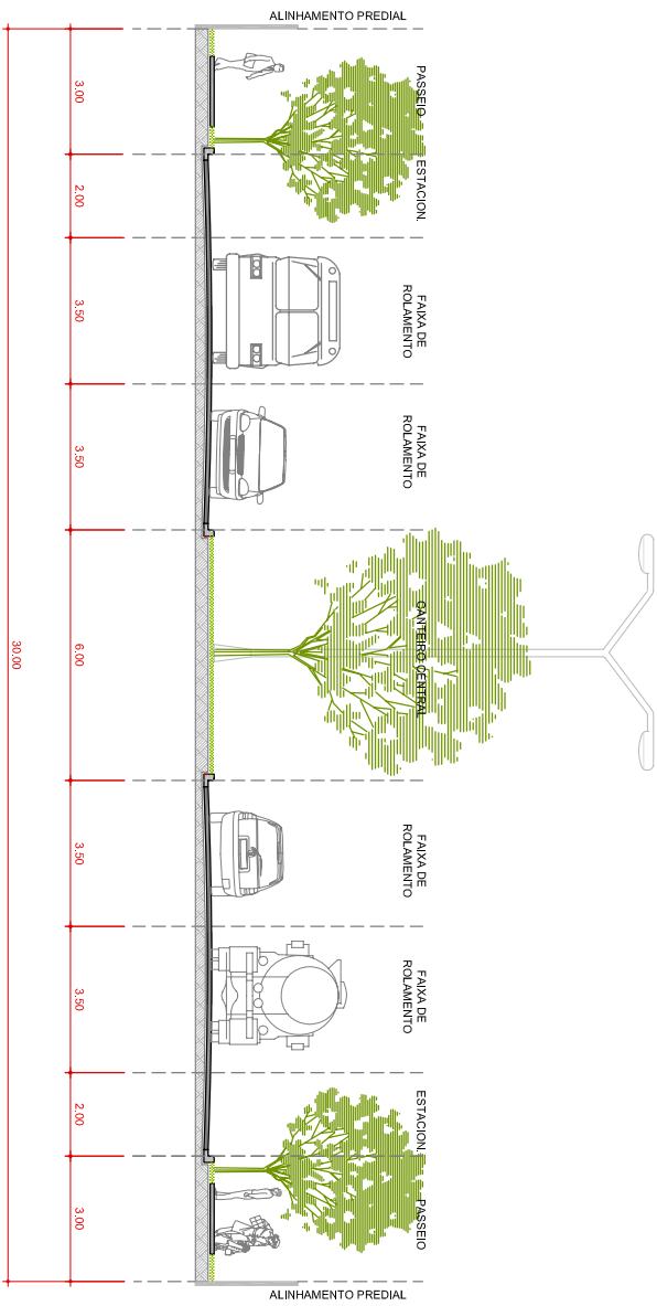
PERFIL VIA ESTRUTURAL ESCALA: 0,00m/1m = 2m ESCALA GRAFICA
