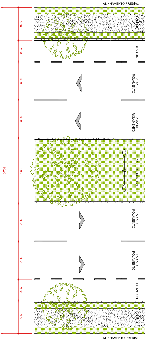
PLANTA VIA ESTRUTURAL ESCALA: 0,00m/1m = 20m ESCALA GRAFICA
