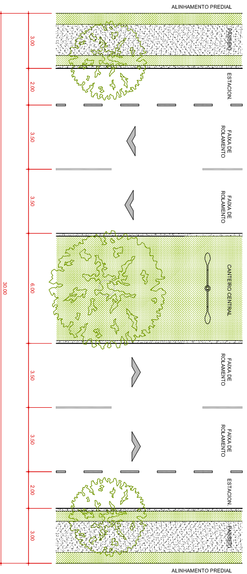
PLANTA VIA ARTERIAL 0,2m = 1,00m em 1m 2m = 3m ESCALA GRAFICA
