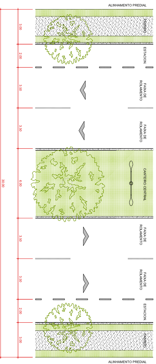
PLANTA VIA ARTERIAL 0,2m = 1,00m 2m = 3m ESCALA GRAFICA
