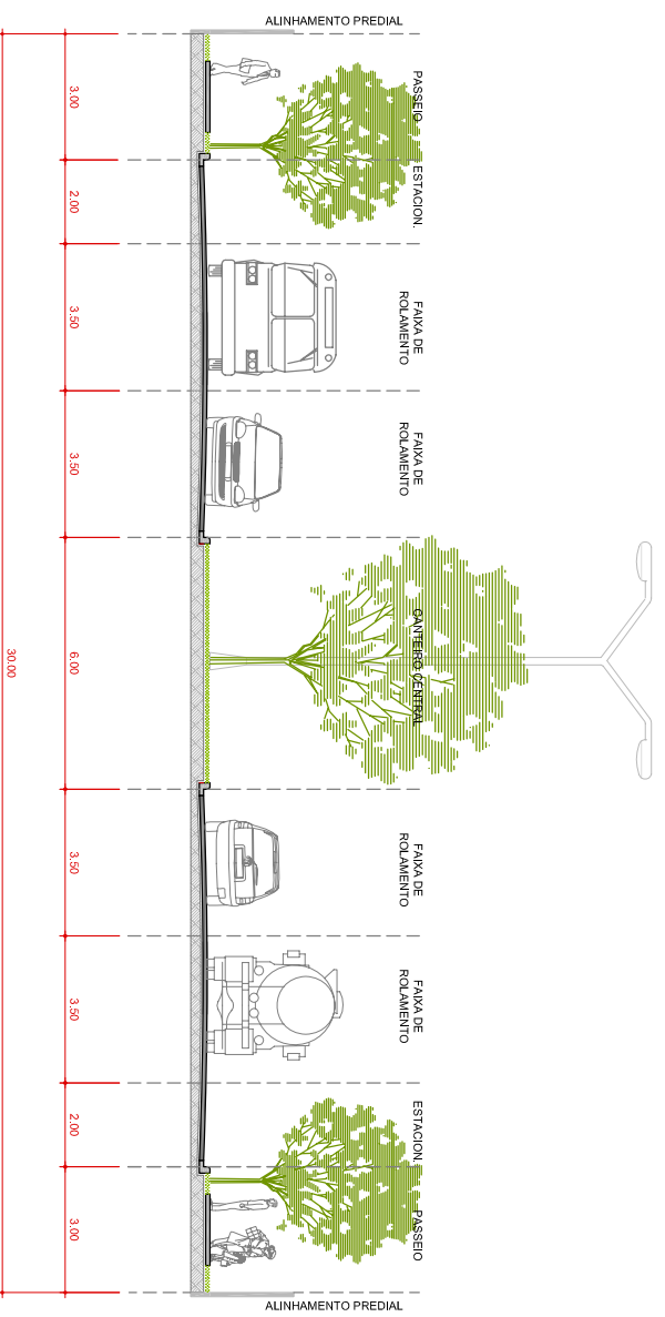
PERFIL VIA ARTERIAL 0,2m = 1,00m 2m = 3m ESCALA GRAFICA
