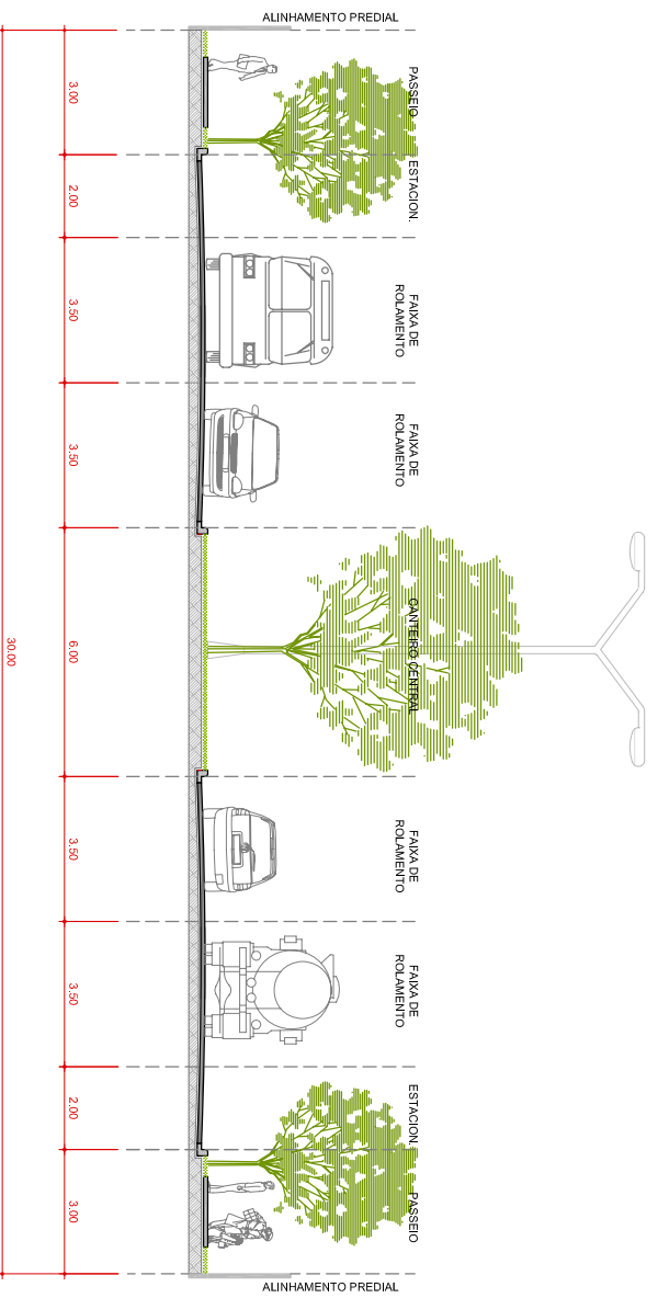
PERFIL VIA ARTERIAL 0,2m = 1,00m em 1m 2m = 3m ESCALA GRAFICA
